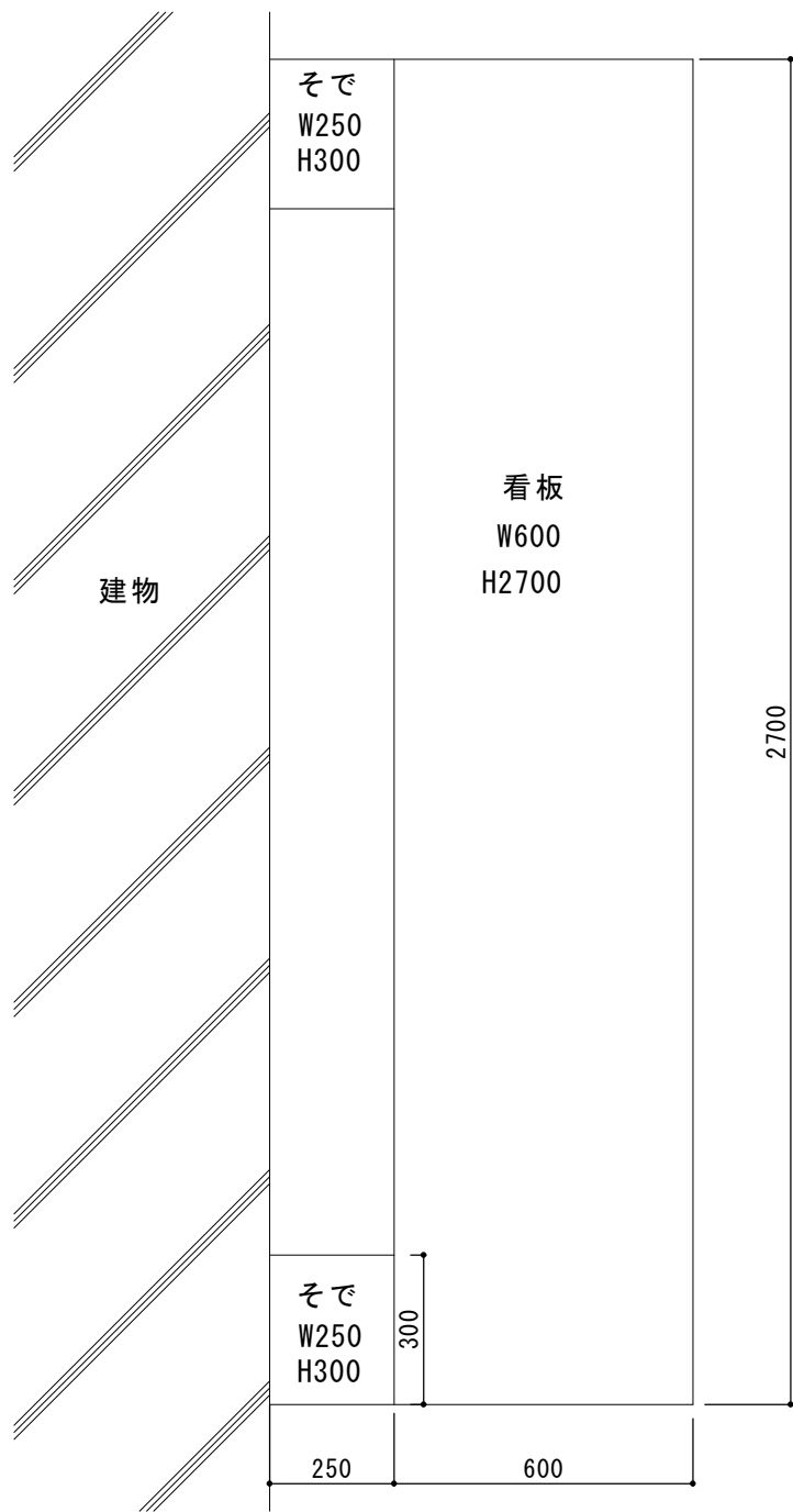
正面図
